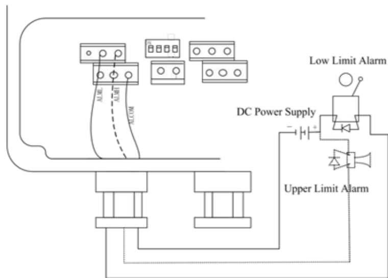
Fig.4.4 (d) Connection of alarm output
